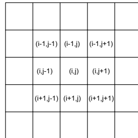
Gambar 3 Cellular automata dua dimensi.
