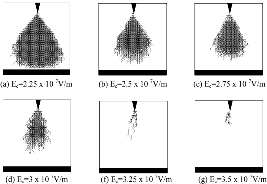
Gambar 11 Pemohonan listrik pada tegangan 20 kV untuk berbagai material dengan medan kritis berbeda.
