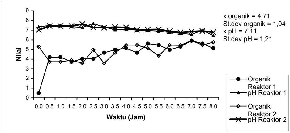
Gambar 9 Fluktuasi kandungan zat organik dan pH pada outlet clarifier pada debit 0,1 L/dtk.
