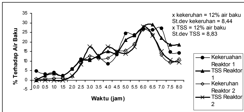
Gambar 8 Fluktuasi kekeruhan dan TSS pada outlet clarifier pada debit 0,1 L/dtk.
