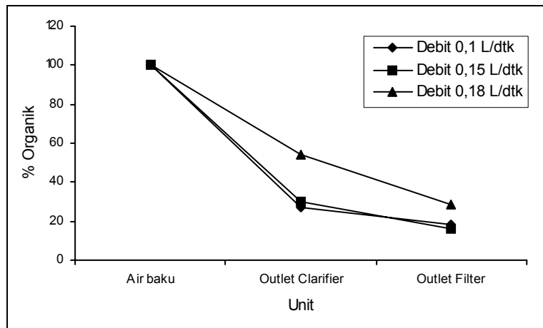
Gambar 4 Grafik penyisihan zat organik pada berbagai variasi debit.
