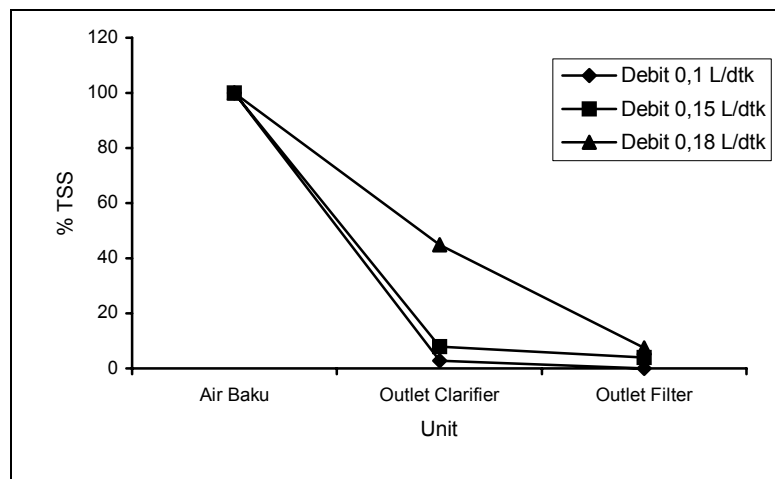
Gambar 2 Grafik penyisihan TSS pada berbagai variasi debit.
