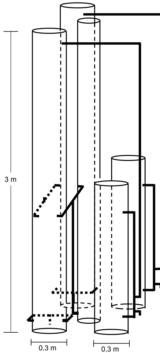
Gambar 14 Instalasi Media Berbutir Skala 1:20.
