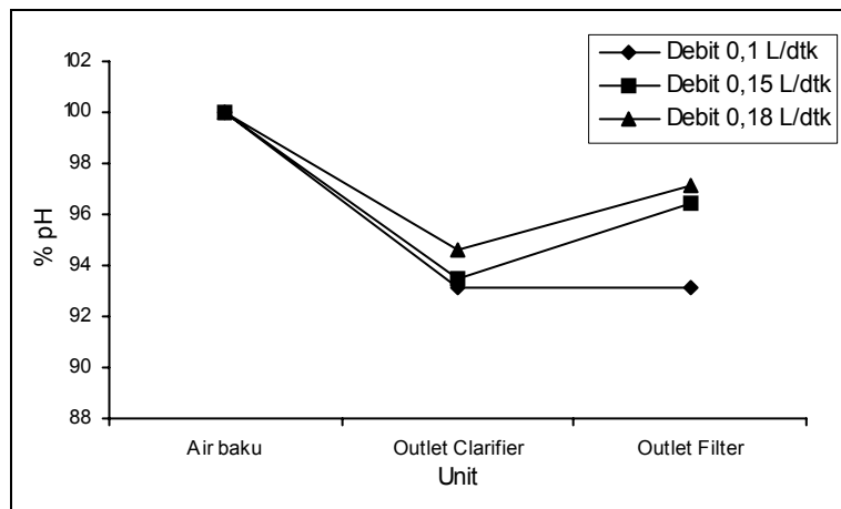
Gambar 5 Grafik fluktuasi pH pada berbagai variasi debit.
