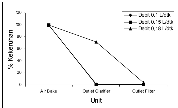
Gambar 3 Grafik penyisihan kekeruhan pada berbagai variasi debit.
