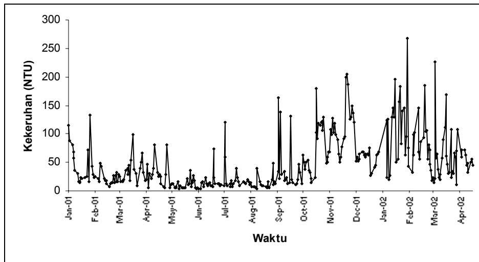
Gambar 1 Fluktuasi kekeruhan air baku PDAM Badak Singa.
