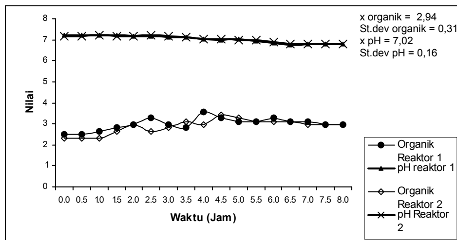
Gambar 13 Fluktuasi zat organik dan pH terhadap waktu pada outlet filter pada debit 0,1 L/dtk.
