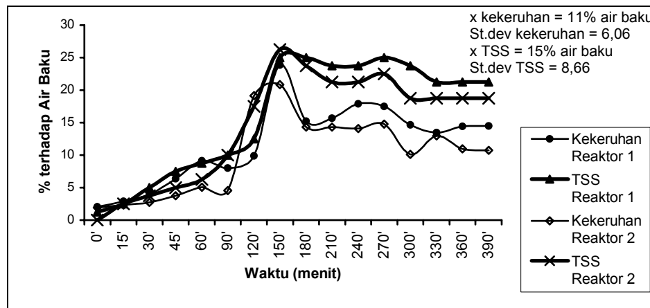
Gambar 10 Fluktuasi kekeruhan dan TSS terhadap waktu pada outlet clarifier pada debit 0,15 L/dtk.
