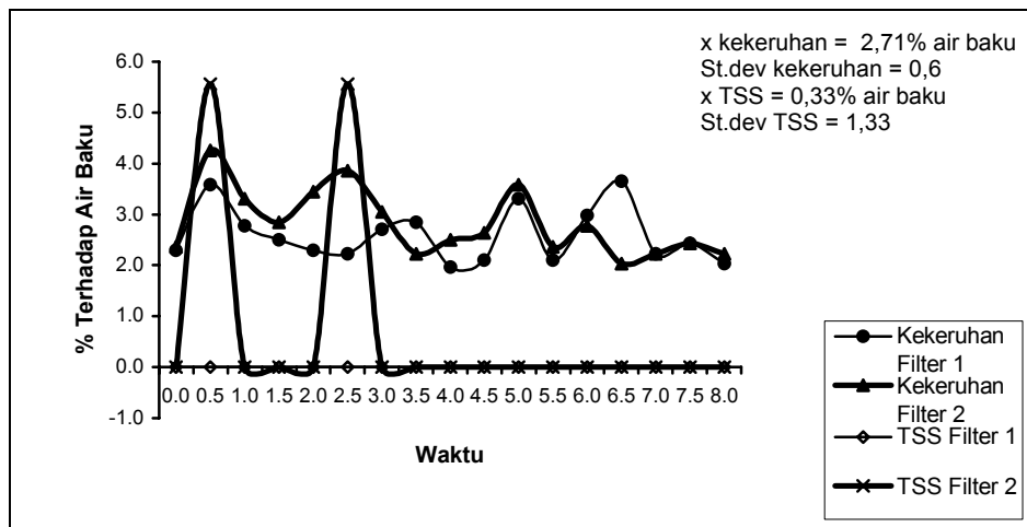
Gambar 12 Fluktuasi kekeruhan dan TSS terhadap waktu pada outlet filter pada debit 0,1 L/dtk.
