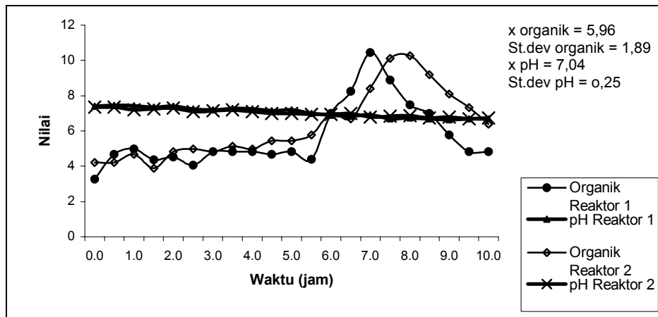
Gambar 7 Fluktuasi zat organik dan pH terhadap waktu pada outlet clarifier pada debit 0,05 L/dtk.
