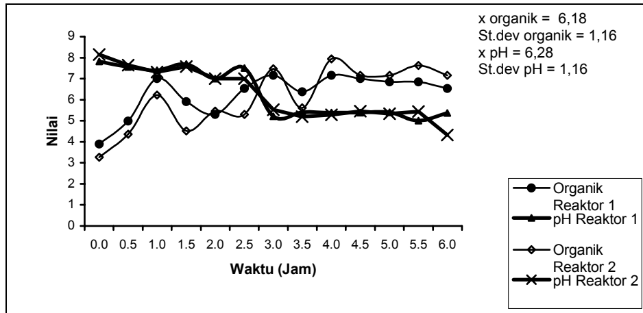
Gambar 11 Fluktuasi zat organik dan pH terhadap waktu pada outlet clarifier pada debit 0,15 L/dtk.
